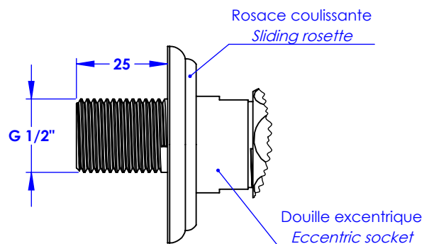
DÉTAIL A ECHELLE 1 : 1.5
